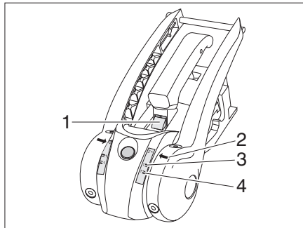
Rys. 152 Kontrola zużycia okładzin ciernych
