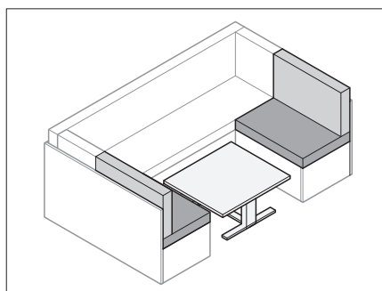
Rys. 68 Przebudowa stołu
