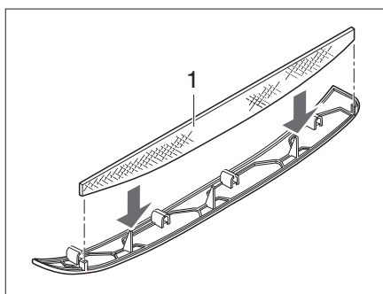
Rys. 156 Filtr kłaczków w klimatyzacji
