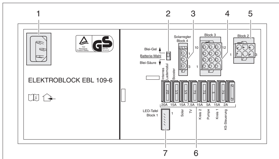
Rys. 93 Blok elektryczny EBL 109
