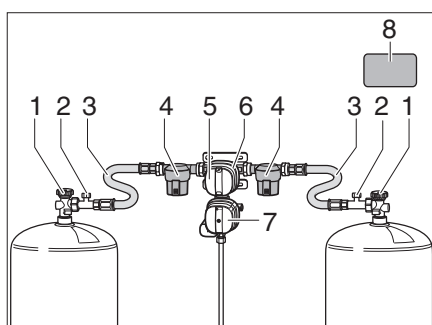
Rys. 85 System przełączający DuoControl
