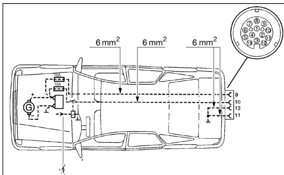
Rys. 102 Schemat instalacyjny samochodu ciągnącego
