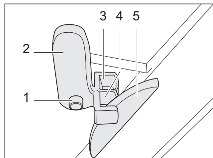
Rys. 51 Okno dachowe Heki w położeniu wentylacyjnym 1
