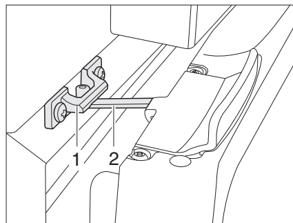
Rys. 136 Drzwi lodówki w położeniu wentylacji (Thetford)
