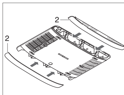
Rys. 157 Panele klimatyzacji
