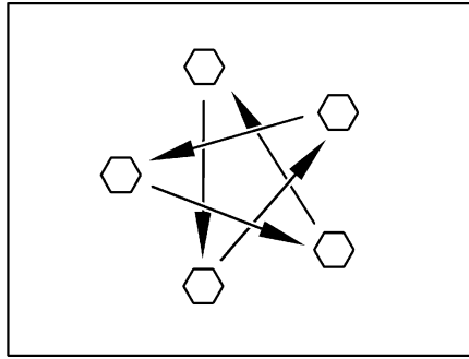
Rys. 160 Nakrętki lub śruby w kołach dokręcać na krzyż.
