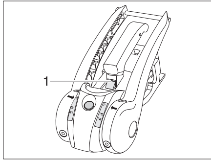
Rys. 153 Wskaźnik zużycia
