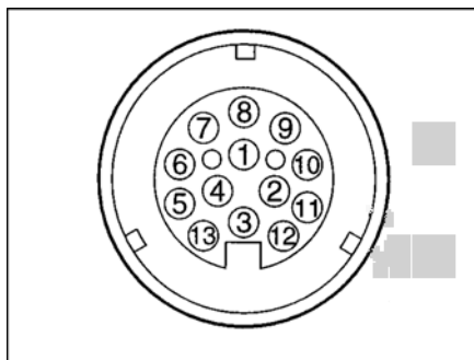
Rys. 101 Widok gniazdka pojazdu ciągnącego (system trzynastobiegunowy Jaeger wg DIN EN 1648-1)
