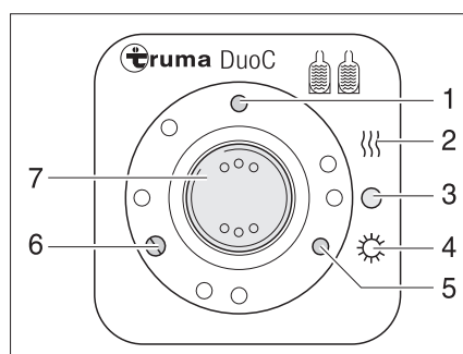
Rys. 86 Panel sterowniczy
