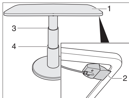
Rys. 56 Stół podnośny kanapy okrągłej
