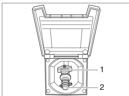
Rys. 84 Zewnętrzne przyłącze gazowe, zamknięty zawór odcinający dopływ gazu
