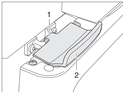
Rys. 135 Blokada drzwi lodówki, zamknięta (Thetford)
