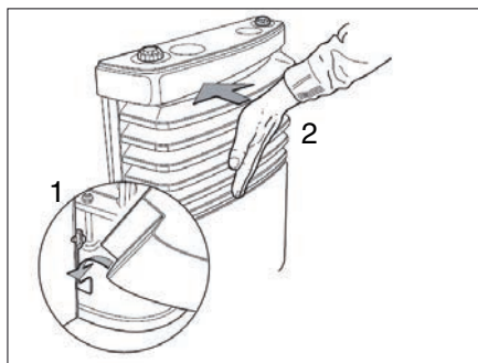
Rys. 108 Mocowanie osłony grzejnika
