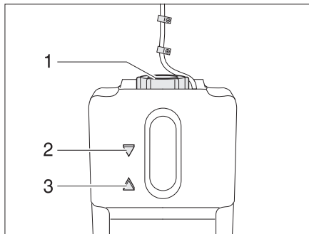
Rys. 154 Zbiornik wyrównawczy grzejnika na wodę ciepłą
