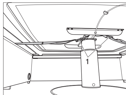
Rys. 57 Zabezpieczenie stołu podnośnego pasami
