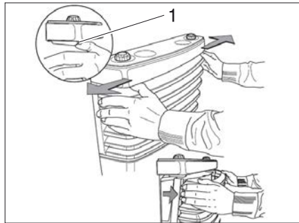
Rys. 106 Zdejmowanie osłony grzejnika
