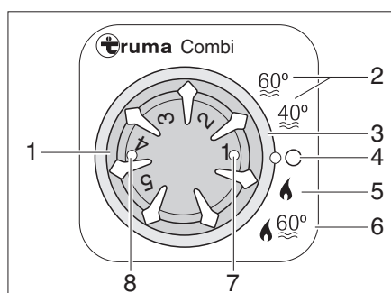
Rys. 113 Panel sterowniczy do grzejnika/bojlera
