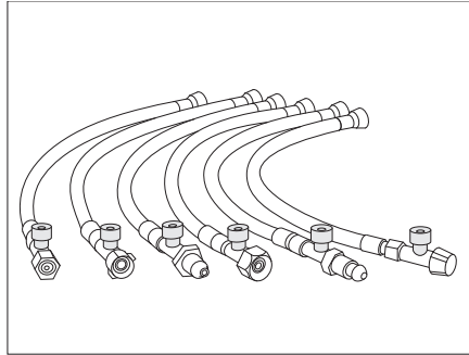
Rys. 235 Wężę wysokociśnieniowe z zabezpieczeniem przed wyciekami gazu w razie uszkodzenia węża (warianty specyficzne dla krajów użytkowników)
