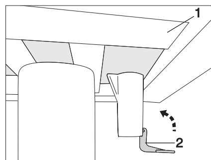
Rys. 98 Blokada stołu jednokolumnowego (odblokowana)
