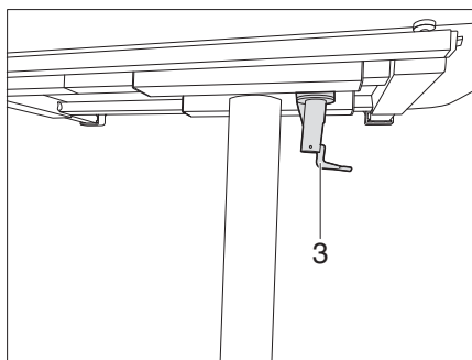
Rys. 115 Ryglowanie stołu składanego
