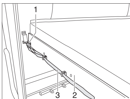
Rys. 168 Łóżko piętrowe (w części tylnej)
