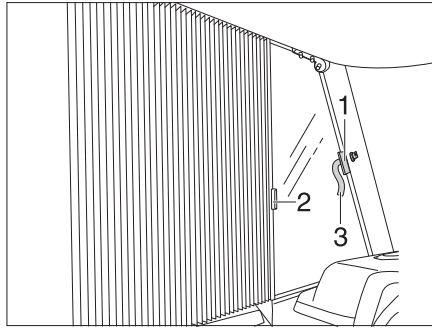
Rys. 12 Zabezpieczanie składanej zasłony zaciemniającej okna kierowcy i pasażera obok kierowcy
