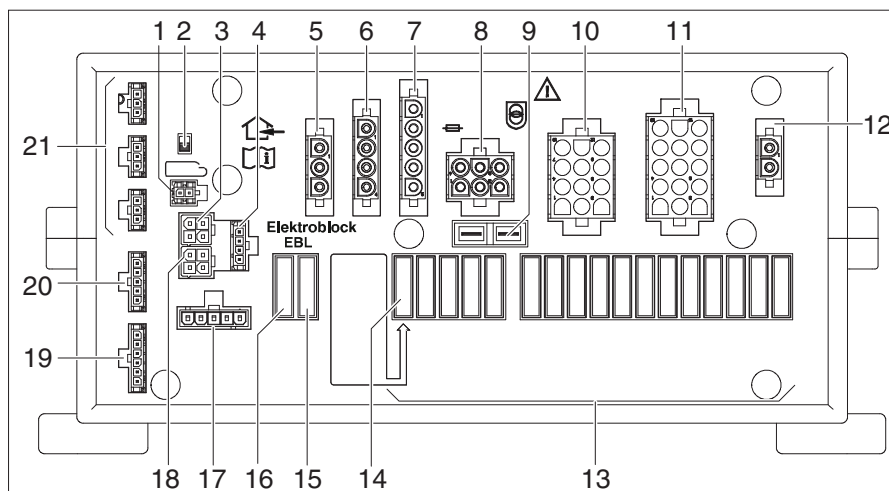
Rys. 243 Blok elektryczny (EBL 402/403)
