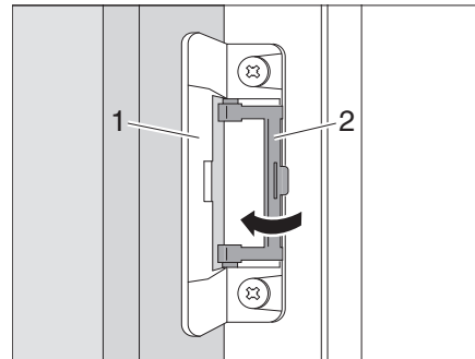
Rys. 331 Blokowanie w położeniu wentylacji
