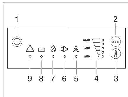
Rys. 322 Elementy obsługowe do lodówki (Dometic seria 10, model RM 10.5)
