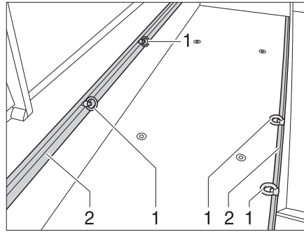
Rys. 2 Zaczepy stabilizacyjne w garażu w tylnej części pojazdu
