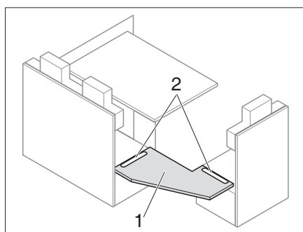
Rys. 176 Mocowanie płyty wzmocniającej
