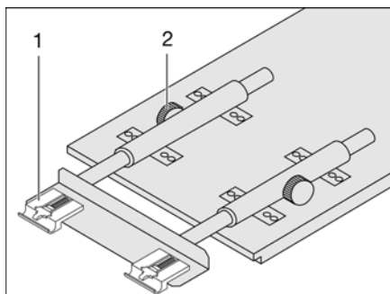
Rys. 91 Powiększanie stołu wiszącego
