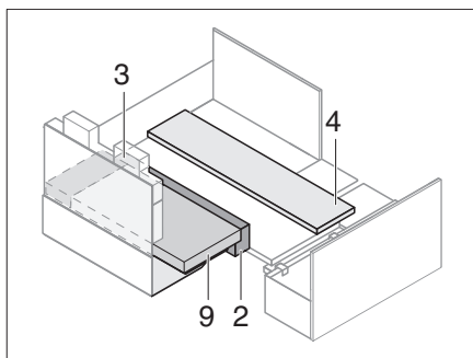
Rys. 218 Pozycjonowanie poduszek dodatkowych
