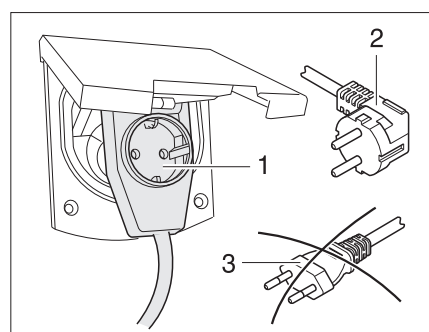
Rys. 284 Podłączenie do złącza kąтового z gniazdkiem
