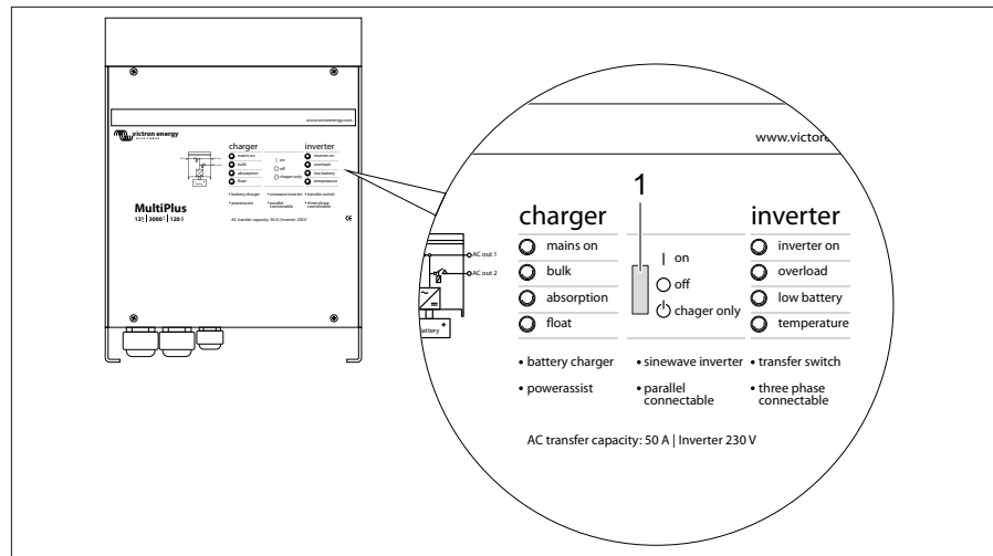
Rys. 238 Falownik MultiPlus
