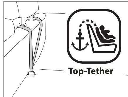
Rys. 20 ISOFIX z systemem Top Tether
