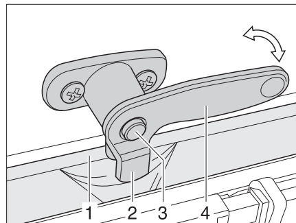
Rys. 69 Dźwignia ryglująca z przyciskiem zabezpieczającym w położeniu „stała wentylacja”
