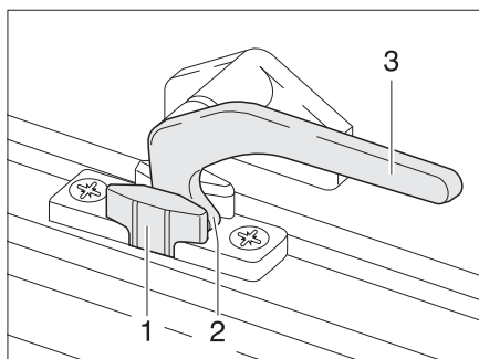
Rys. 68 Dźwignia ryglująca w położeniu „stała wentylacja”
