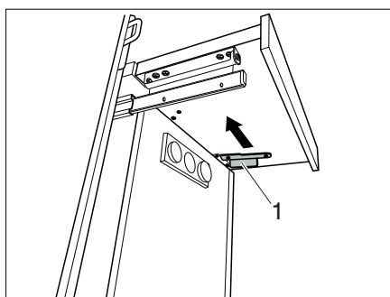
Rys. 130 Zabezpieczanie poszerzenie
