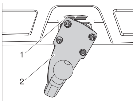
Rys. 4 Hak holowniczy
