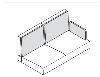
Rys. 206 Poduszki do nakładek pod plecy
