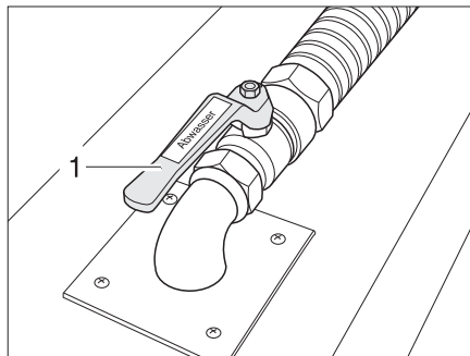
Rys. 338 Zawór kurkowy ściekowy
