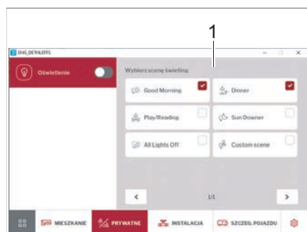
Rys. 259 Podmenu PRYWATNE
