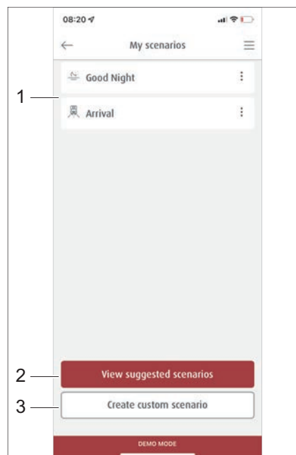
Rys. 278 Zarządzanie scenariuszami
