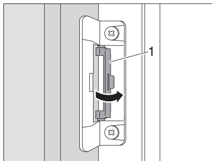
Rys. 332 Przekręcanie blokady z powrotem do położenia wyjściowego
