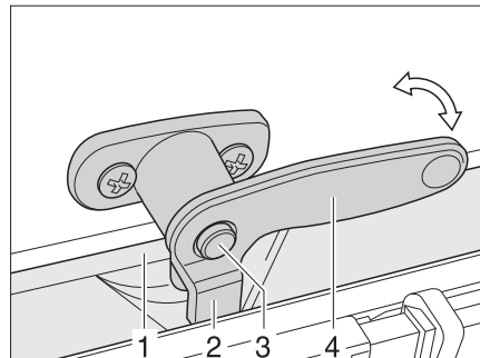
Rys. 71 Dźwignia ryglująca z przyciskiem zabezpieczającym w położeniu „zamknięta”
