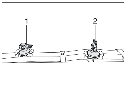
Rys. 343 Zawór kurkowy spustowy
