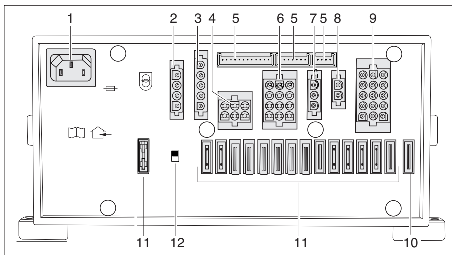
Rys. 240 Blok elektryczny (EBL 111)
