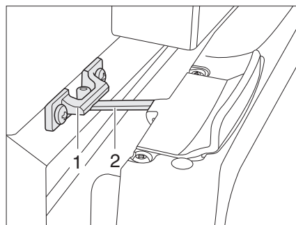
Rys. 329 Drzwi lodówki w położeniu wentylacji (Thetford)
