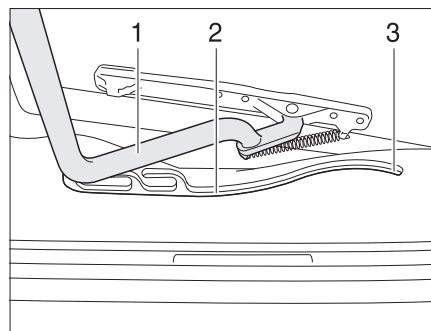
Rys. 86 Okno dachowe Heki, prowadnica
