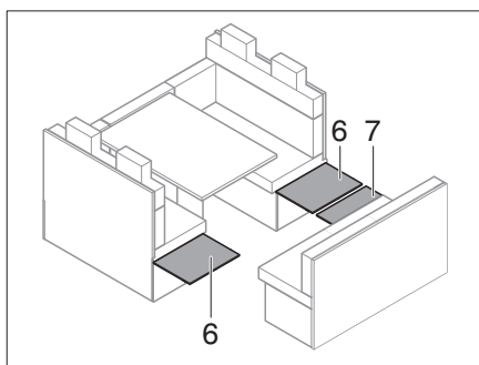
Rys. 216 Rozkładanie ścian bocznych
