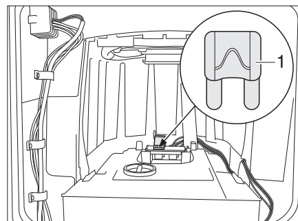
Rys. 288 Bezpiecznik toalety Thetford (alternatywa)
