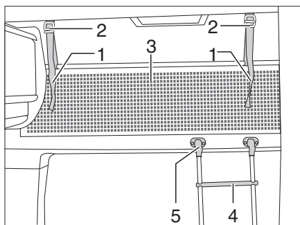
Rys. 148 Łóżko w alkowie
