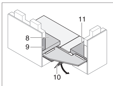
Rys. 178 Podparcie płyty wzmocniającej
