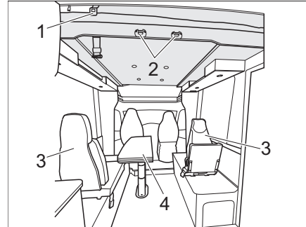
Rys. 159 Łóżko podnoszone elektrycznie (wariant 3)
