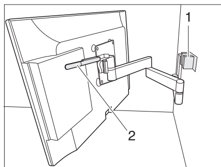
Rys. 9 Mocowanie z ramieniem przegubowym
