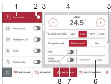
Rys. 260 Grzejnik
