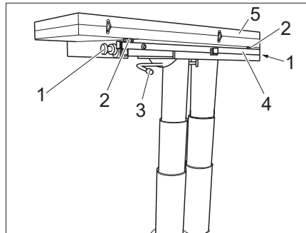
Rys. 110 Powiększanie stołu
