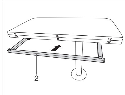
Rys. 114 Wsuwanie podstawy stołu składanego
