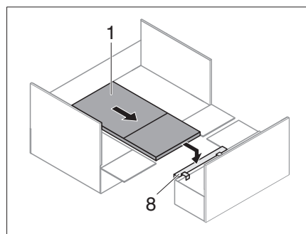
Rys. 217 Stół na podkładce skrzyni łóżka
