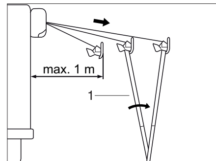
Rys. 36 Rozstawianie markizy
