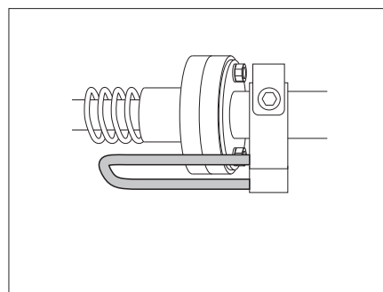
Rys. 147 Dźwignia zabezpieczająca w położeniu zabezpieczonym
