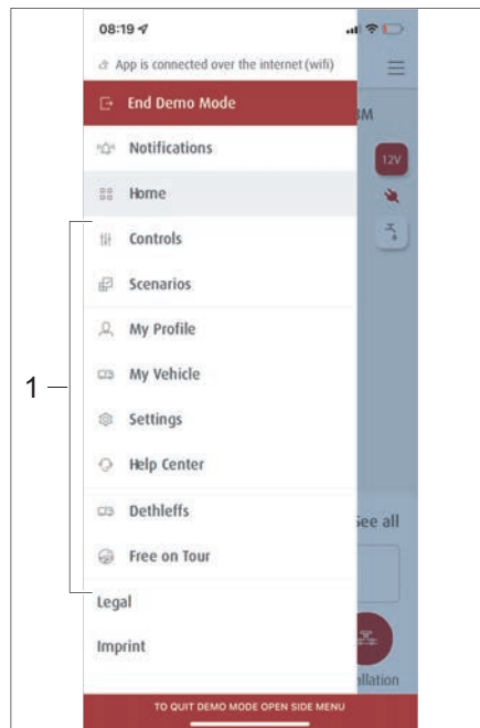
Rys. 276 Podmenu
