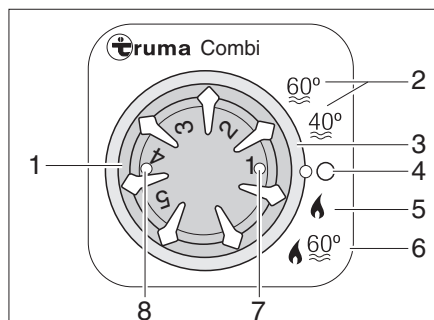
Rys. 293 Panel sterowniczy do grzejnika/bojlera
