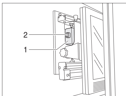
Rys. 8 Mocowanie w szafie na telewizor
