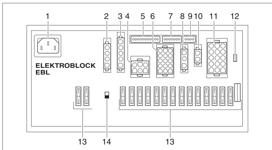
Rys. 242 Blok elektryczny (EBL 102)
